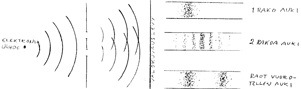
Kuva 1. Kaksoisrakokoe
