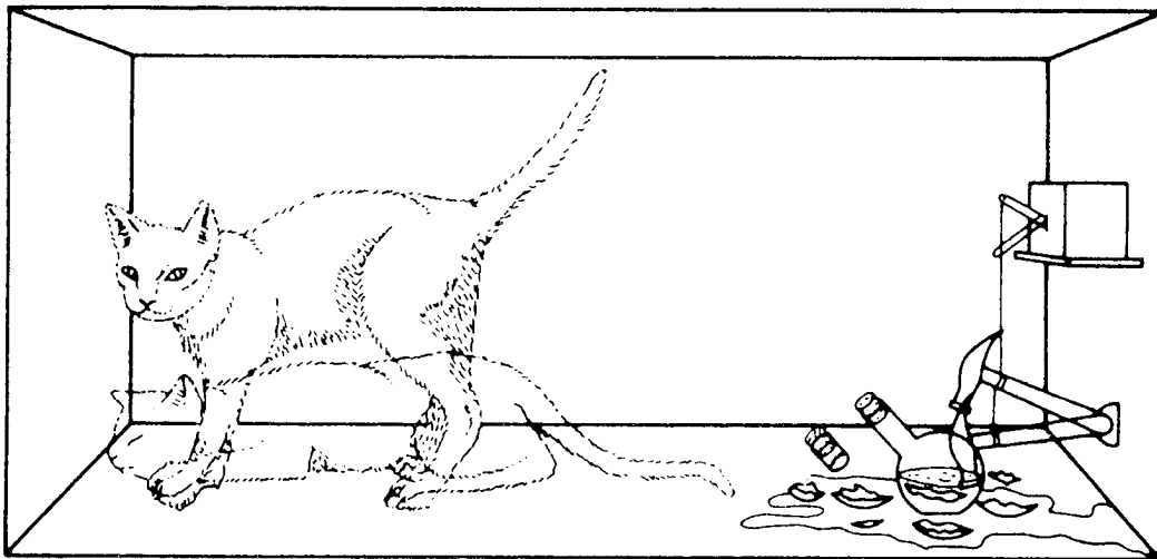
Kuva 2. Schrödingerin kissa
